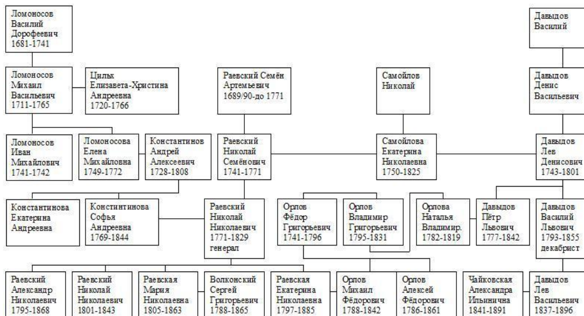
Рис. 3. Смешанная генеалогическая схема (таблица)
